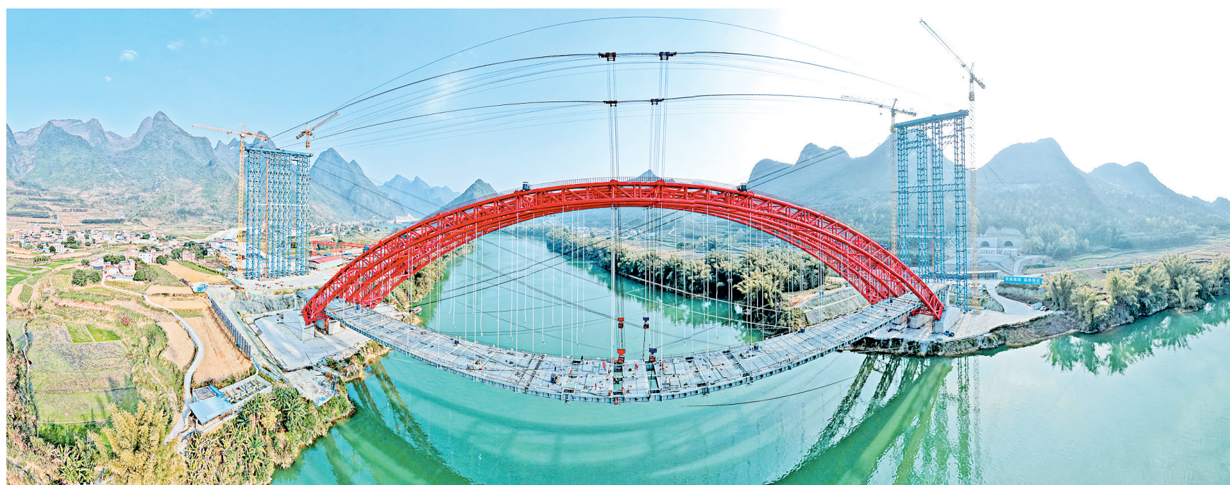
▲3月2日,随着最后合龙口焊接端顺利焊接完成,位于忻城县红渡镇六螺村的来都高速公路全段红水河特大桥右幅桥面格子梁顺利合龙。
